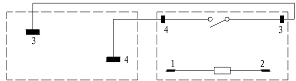
接线图 (Terminal arrangement)
