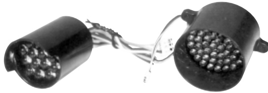
Ø = 26мм BL0102-14-34 красно-зеленый Imkb = 1600+2400 (красный) 1200+2200 (зеленый)
